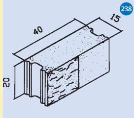
Macizo Liso-split standard
