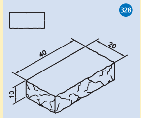
Macizo Split 1/2 alt 2 esquinas
